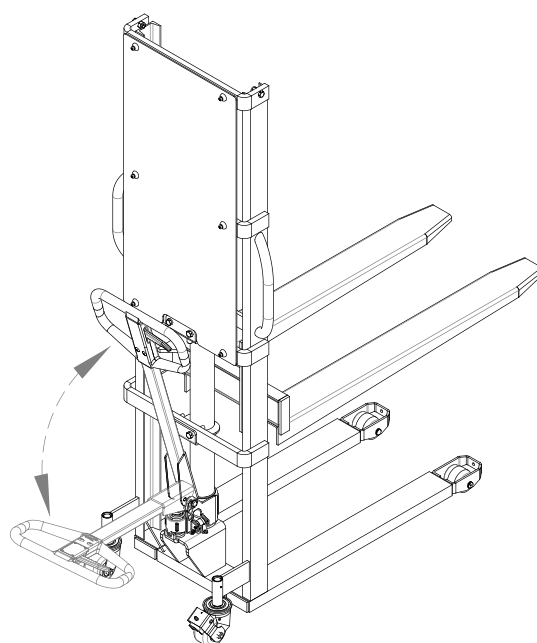
Figura 9 – Bombeamento.
