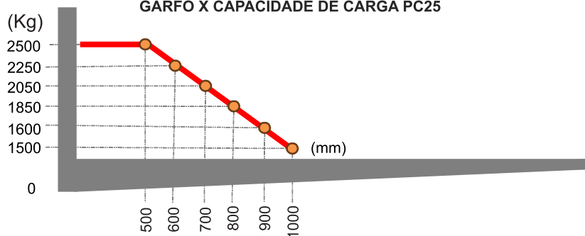
CENTRO DE GRAVIDADE DA CARGA NO GARFO X CAPACIDADE DE CARGA PC25
