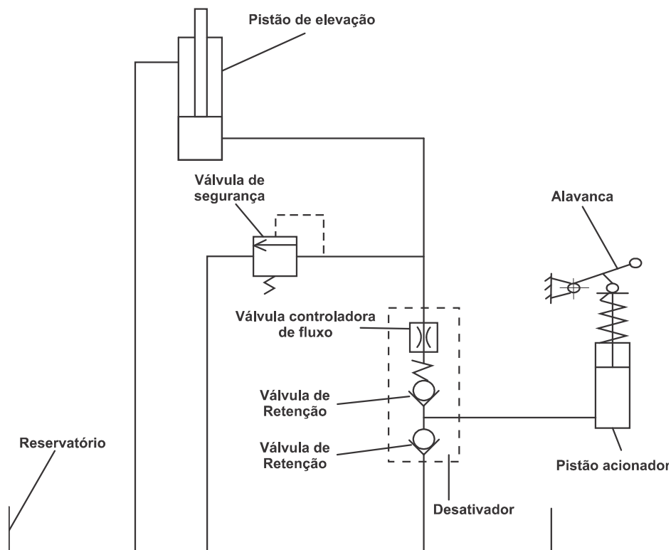
Figura 12 - Circuito hidráulico
