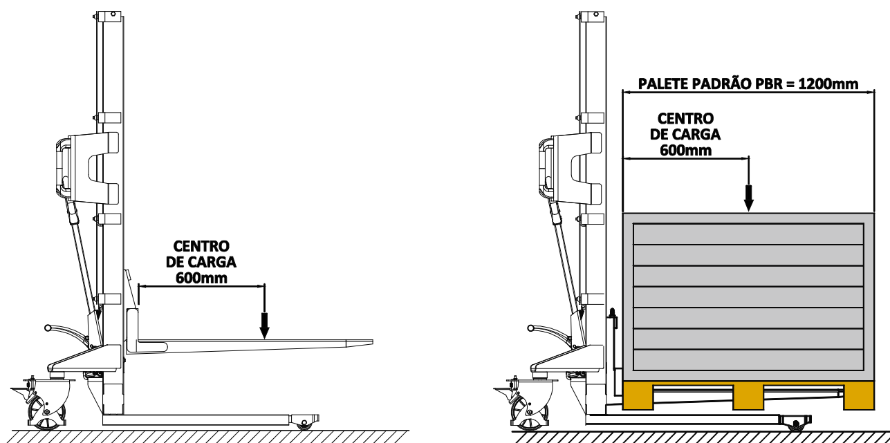
Figura 1 – Centro de carga
